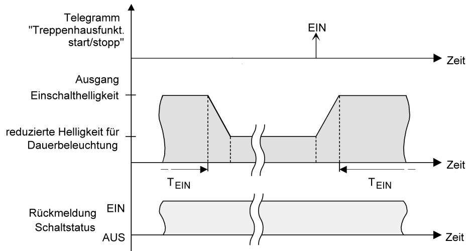
Bild 57: Die Dauerbeleuchtung der Treppenhausfunktion mit Soft-AUS-Funktion
