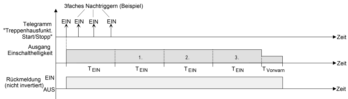
Bild 58: Zeitverlängerung der Treppenhausfunktion
