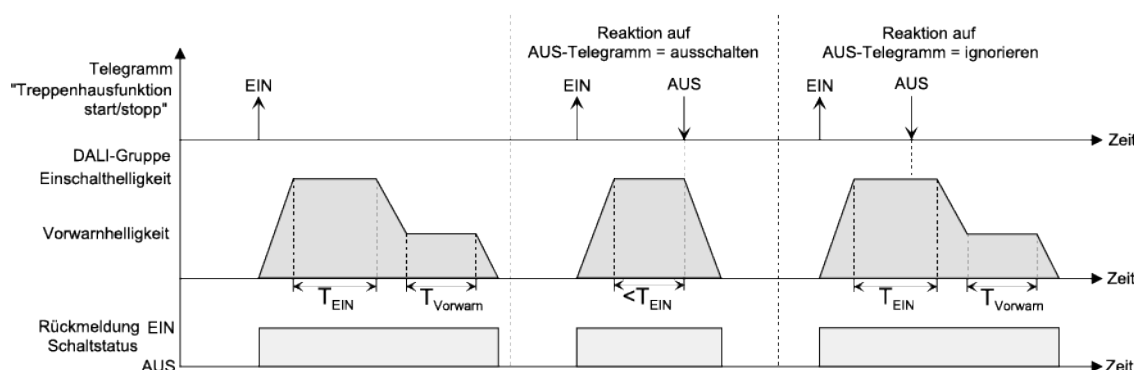
Bild 53: Ausschaltverhalten der Treppenhausfunktion mit Soft-Funktionen (als Beispiel mit Minimalhelligkeit = 0%)
