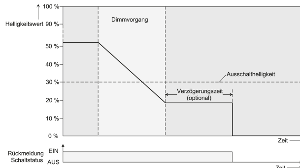
Bild 49: Dimm- und Schaltverhalten der automatischen Ausschaltfunktion
