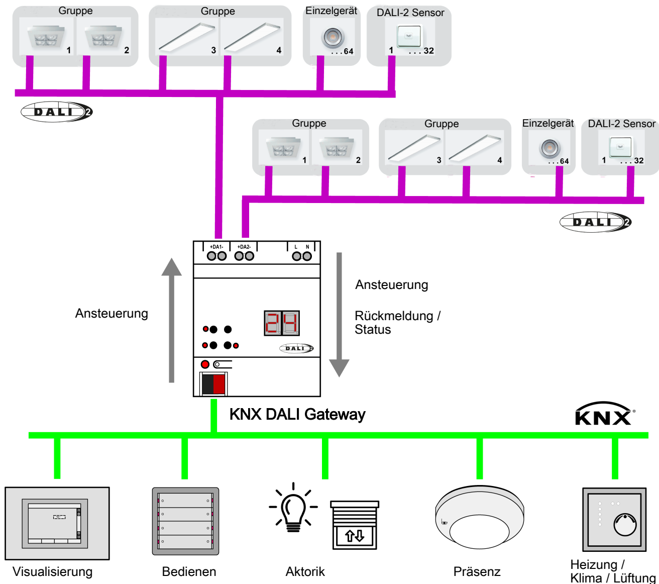
Bild 10: Prinzipübersicht einer KNX DALI Systemanbindung mit DALI Sensoren (Beispiel)
