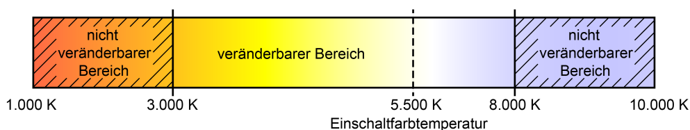
Bild 24: Beispiel eines konfigurierten Farbtemperaturbereichs mit Einschaltfarbtemperatur
