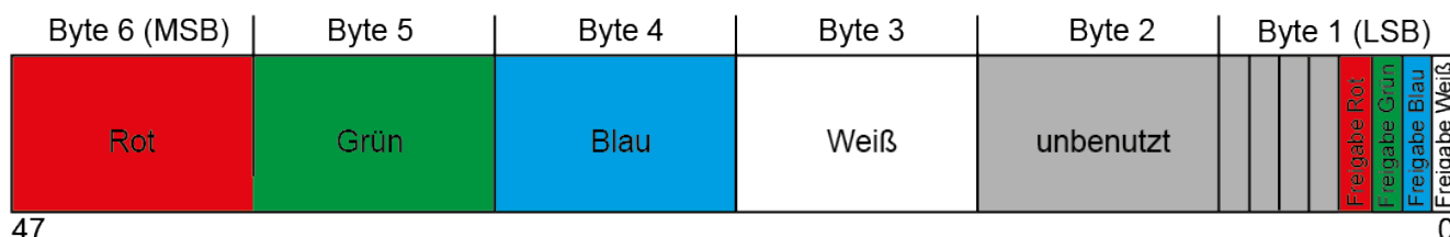
Bild 34: KNX Datentyp "RGBW kombiniert" (DPT 251.600)
