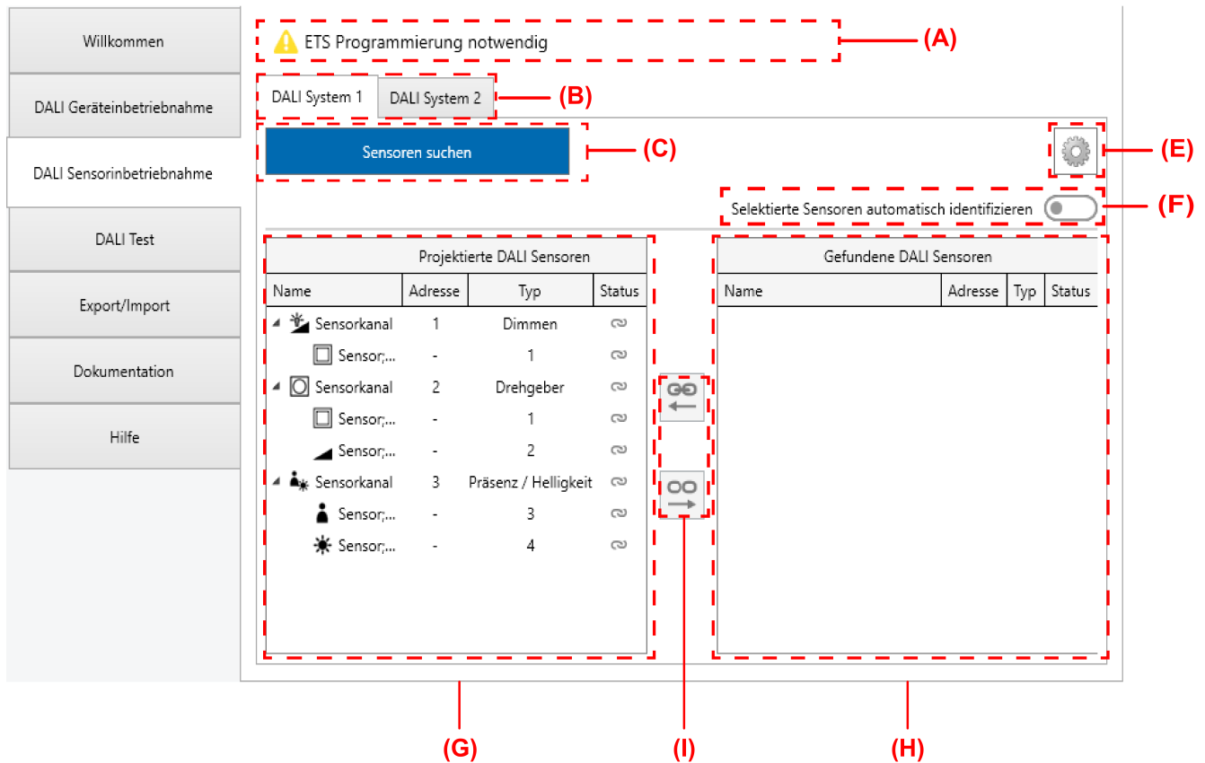
Bild 85: DALI Inbetriebnahmeumgebung in der DCA - Sensoren
