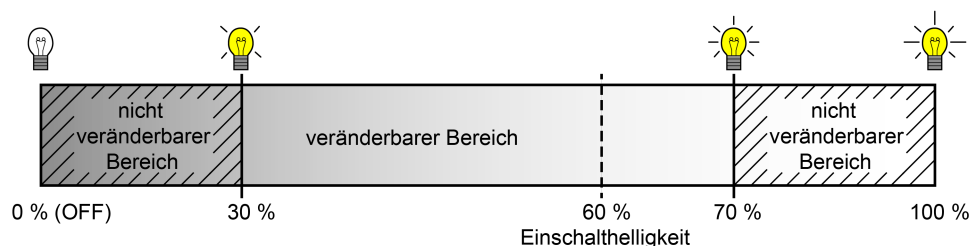
Bild 18: Beispiel eines Helligkeitsbereichs mit Einschalthelligkeit
