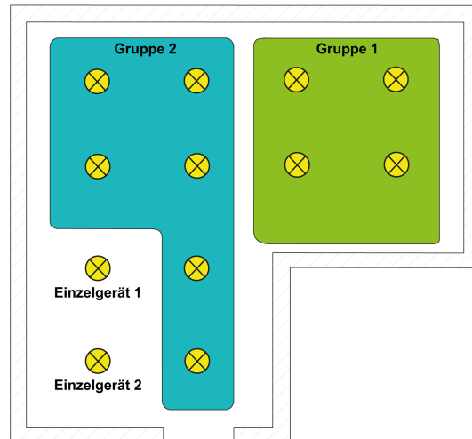
Bild 7: Beispiel einer Gruppen- und Einzelgerätesteuerung
