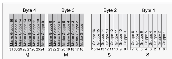
Bild 14: Struktur der Objekte der Sammelrückmeldung am Beispiel des Objekts für die Gruppen 1-16
