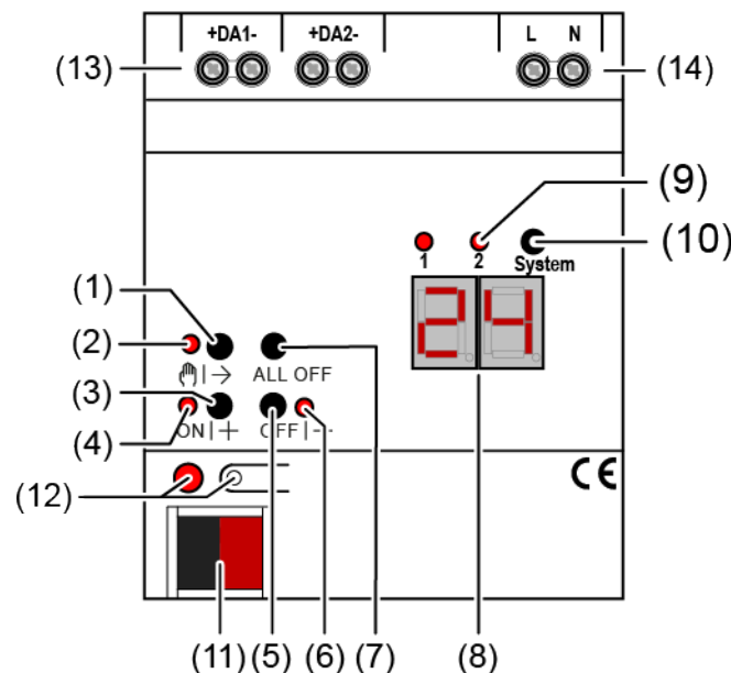
Bild 1: Geräteaufbau
