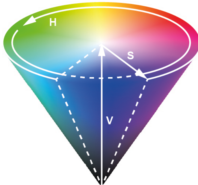
Bild 35: HSV-Farbraum
