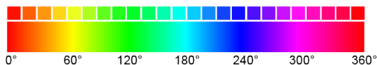
Bild 36: HSV-Farbwinkel (Hue)
