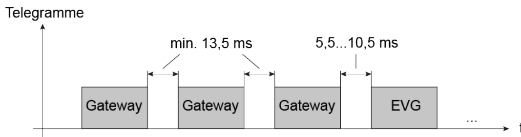
Bild 13: Pausenzeiten zwischen DALI Befehlen
