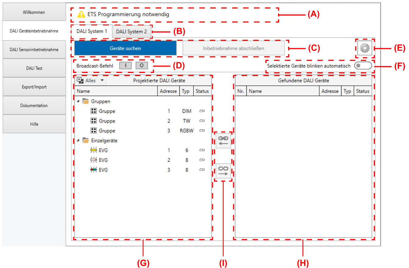
Bild 69: DALI Inbetriebnahmeumgebung in der DCA für Betriebsgeräte
