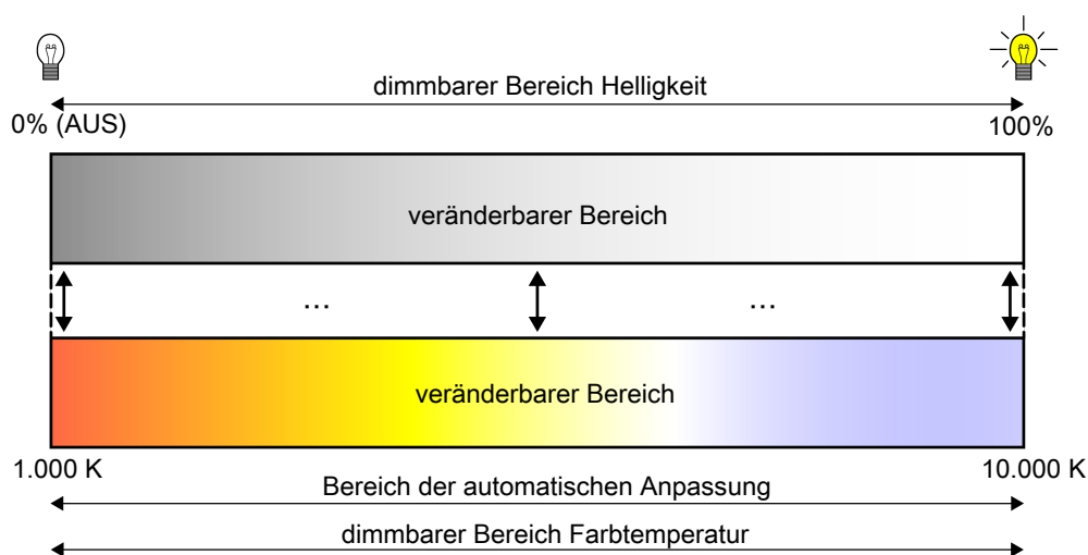
Bild 18: Automatische Anpassung der Farbtemperatur an die eingestellte Helligkeit Beispiel im maximalen Helligkeits- und Farbtemperaturbereich
