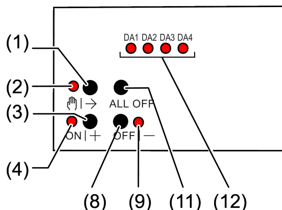
Bild 7: Bedienfeld
