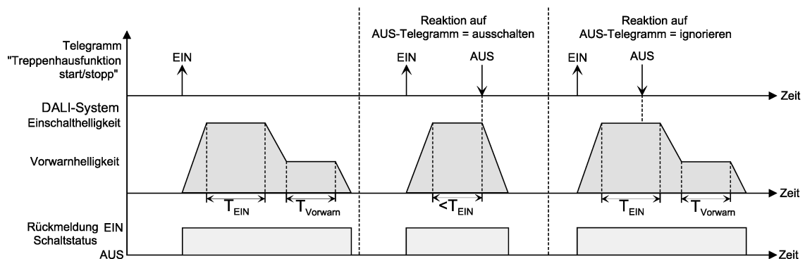
Bild 39: Ausschaltverhalten der Treppenhausfunktion mit Soft-Funktionen (als Beispiel mit Minimalhelligkeit = 0%)
