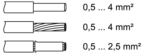
Bild 3: Klemmbare Leiterquerschnitte
