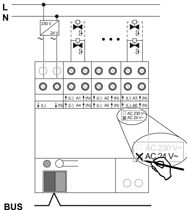
图像 3: 24 V 伺服驱动装置接口
