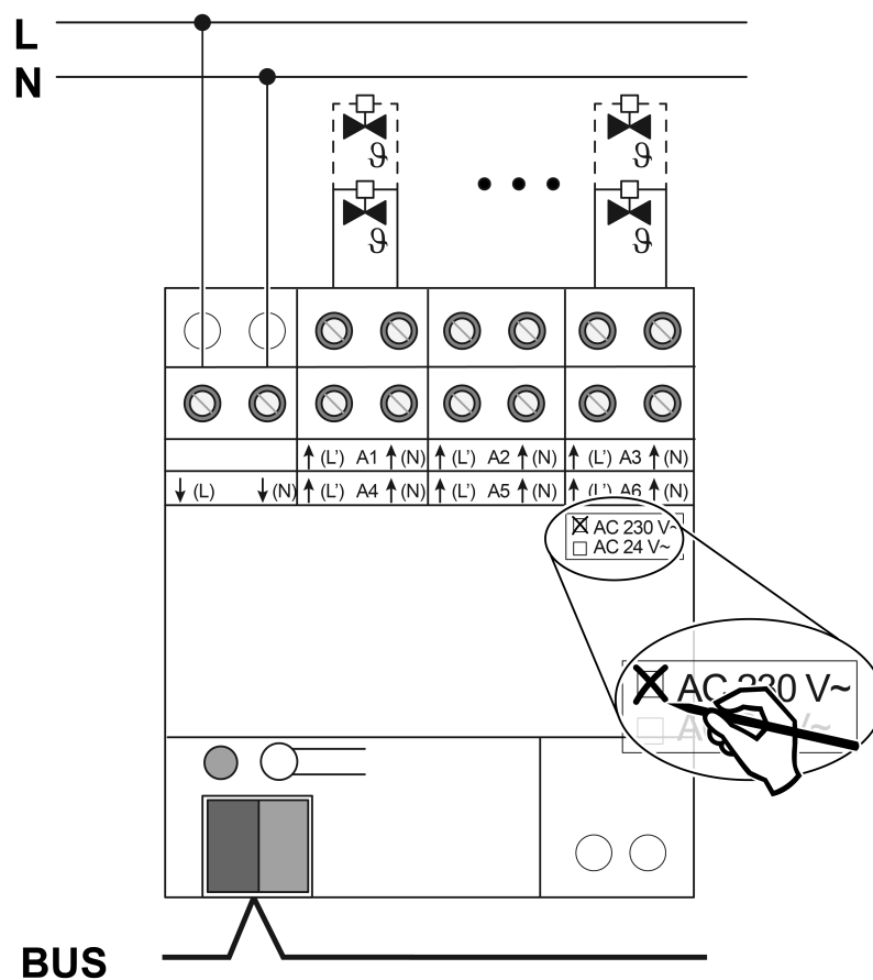
图像 2: 230 V 伺服驱动装置接口
