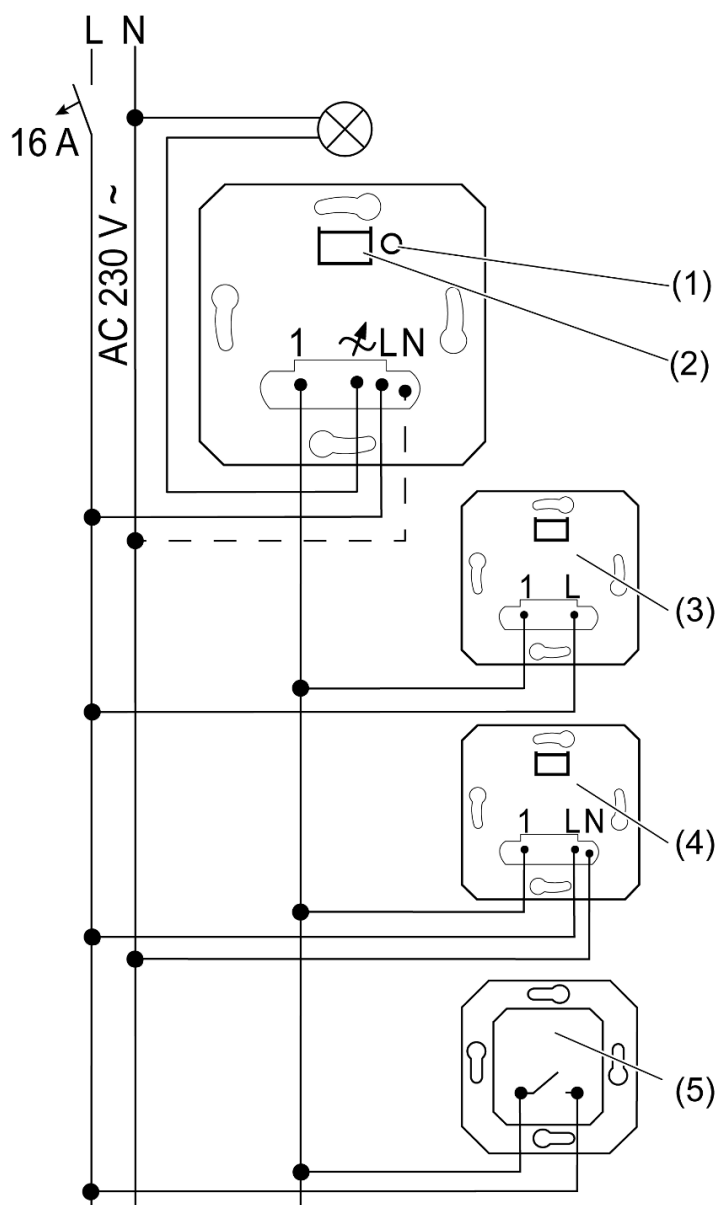
图像 1: 含有可选分机的接线图
