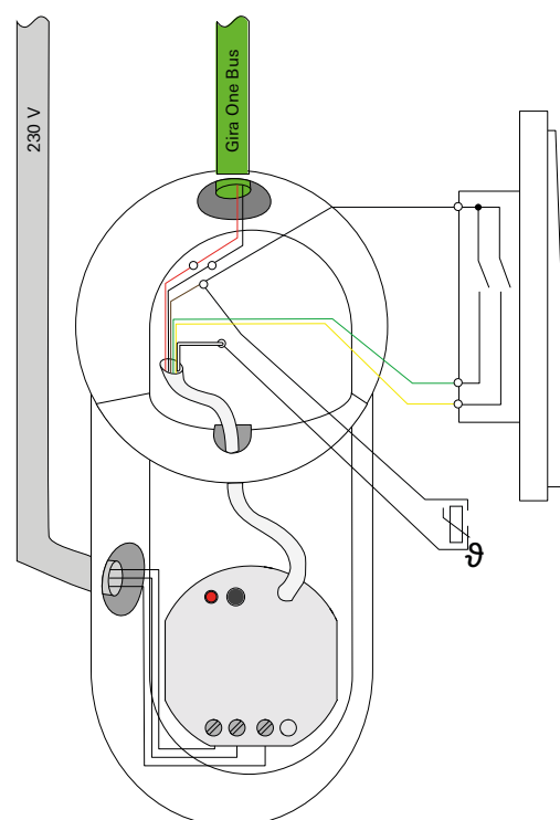
Elektroniczna puszka instalacyjna ze stałą ścianką działową
