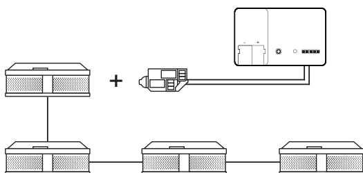
Łączenie w sieć czujników alarmowych dymu Gira
