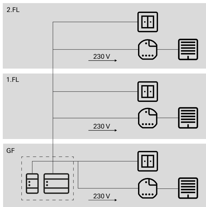
Decentralna instalacja aktorów
